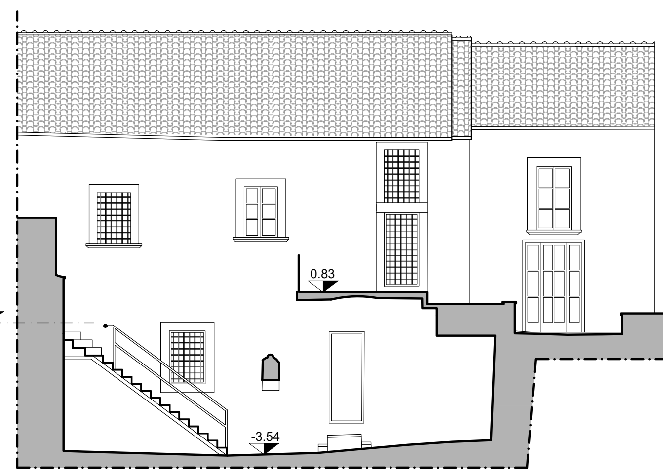
SEZIONE D-D'
