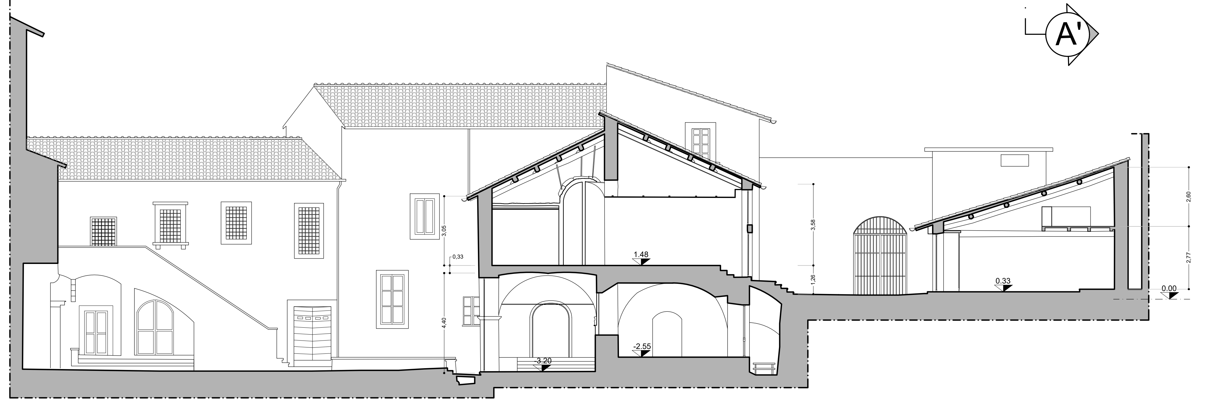
SEZIONE A-A'
