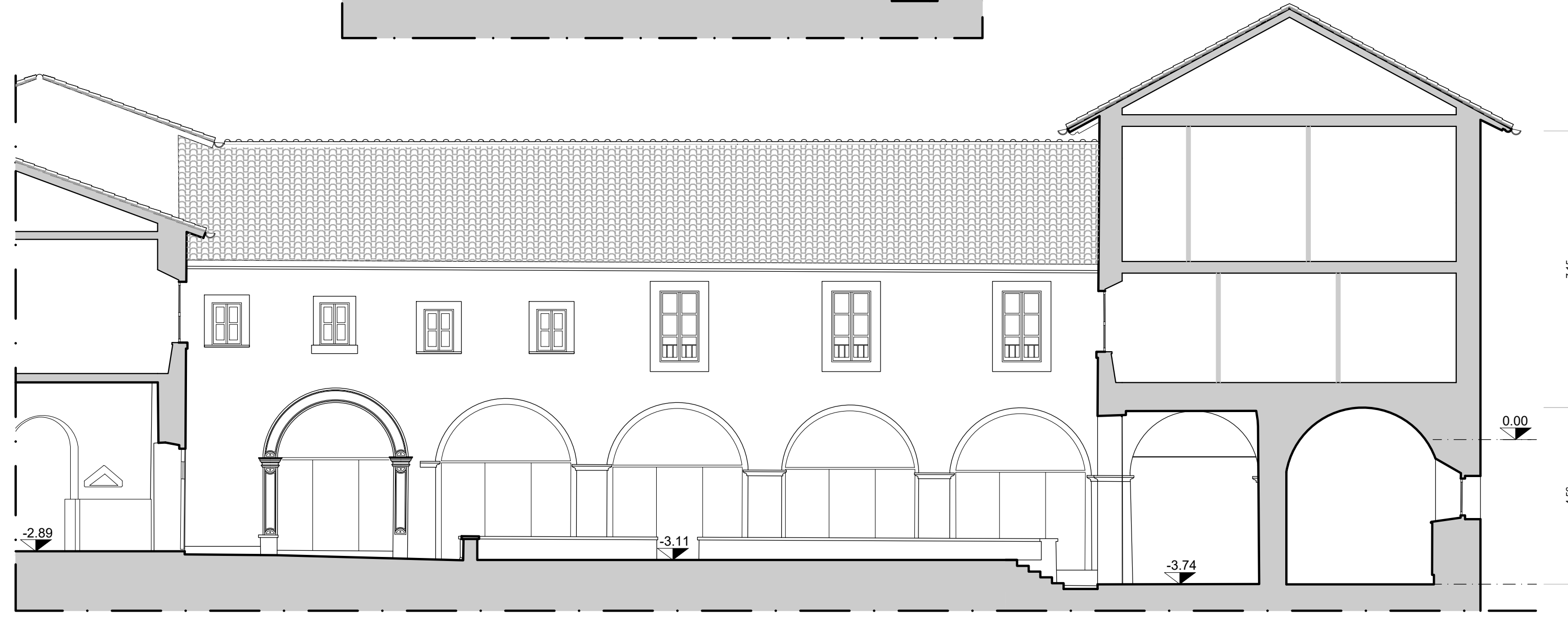
SEZIONE B-B'
