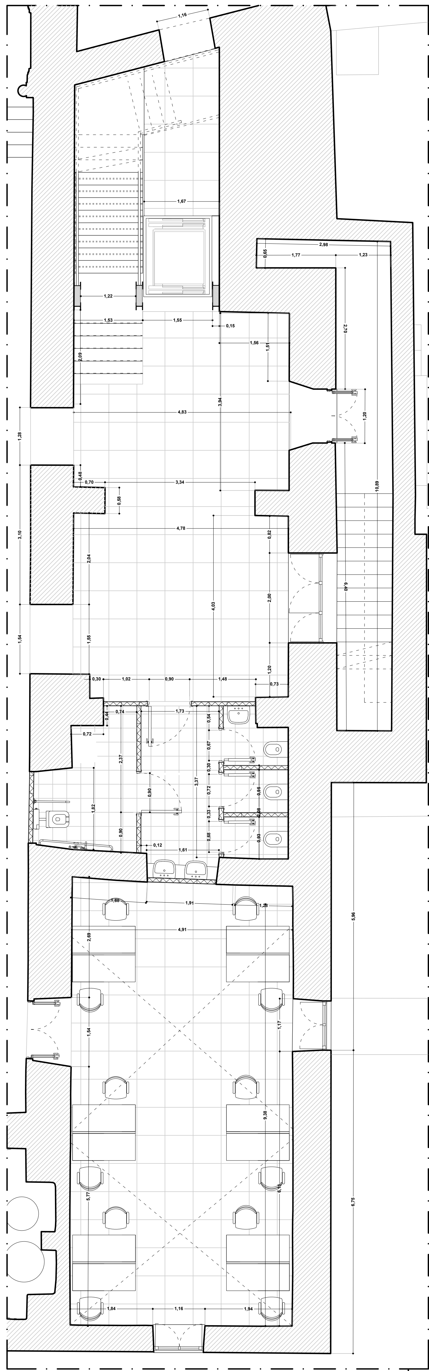
Pianta Atrio ingresso T.4-T.5 - Aula T.11
