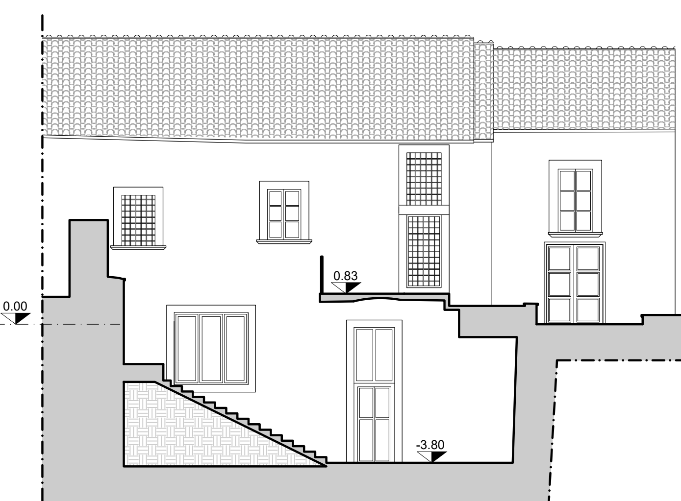
SEZIONE D-D'
