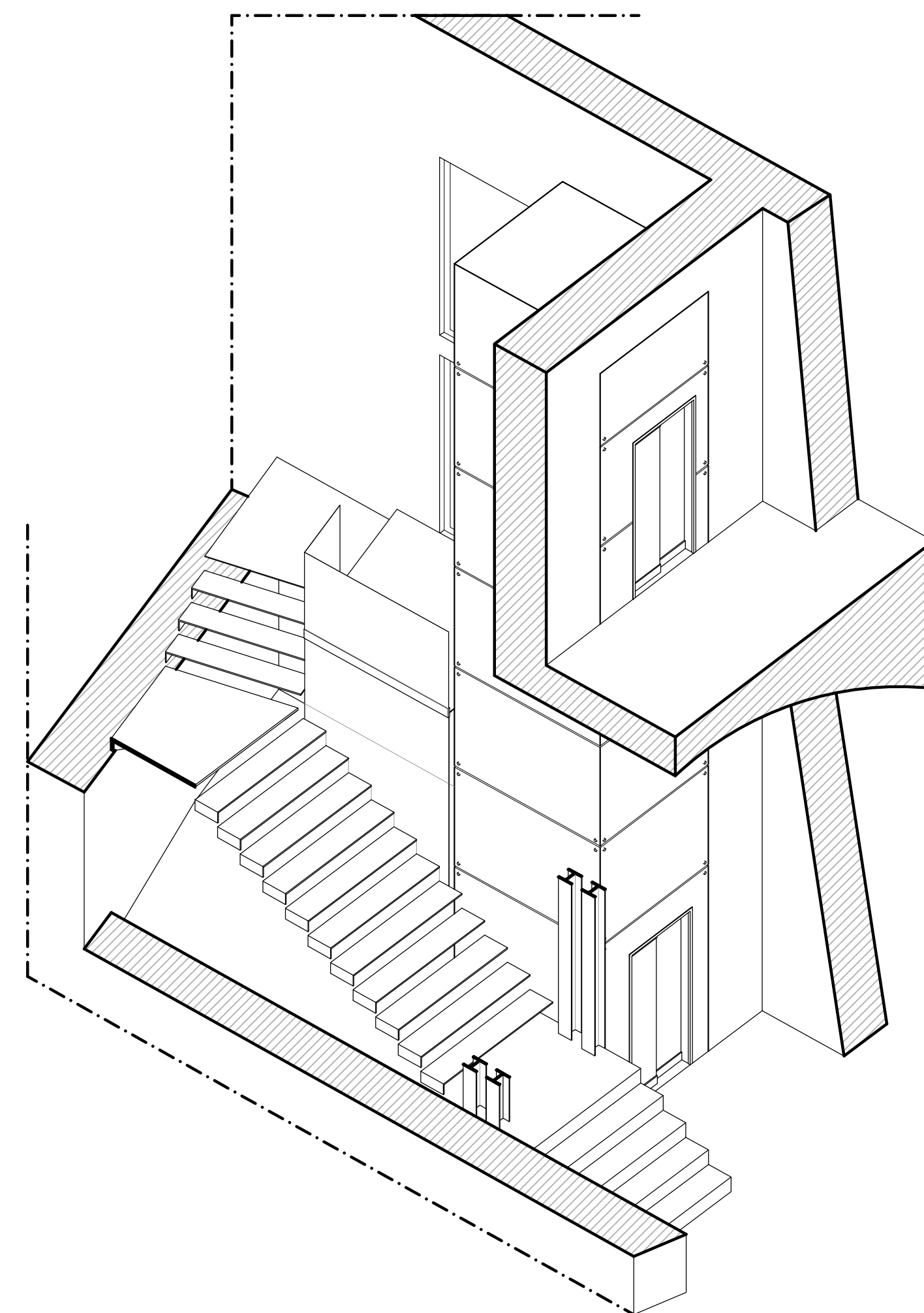
SPACCATI ASSONOMETRICI VANO SCALA
