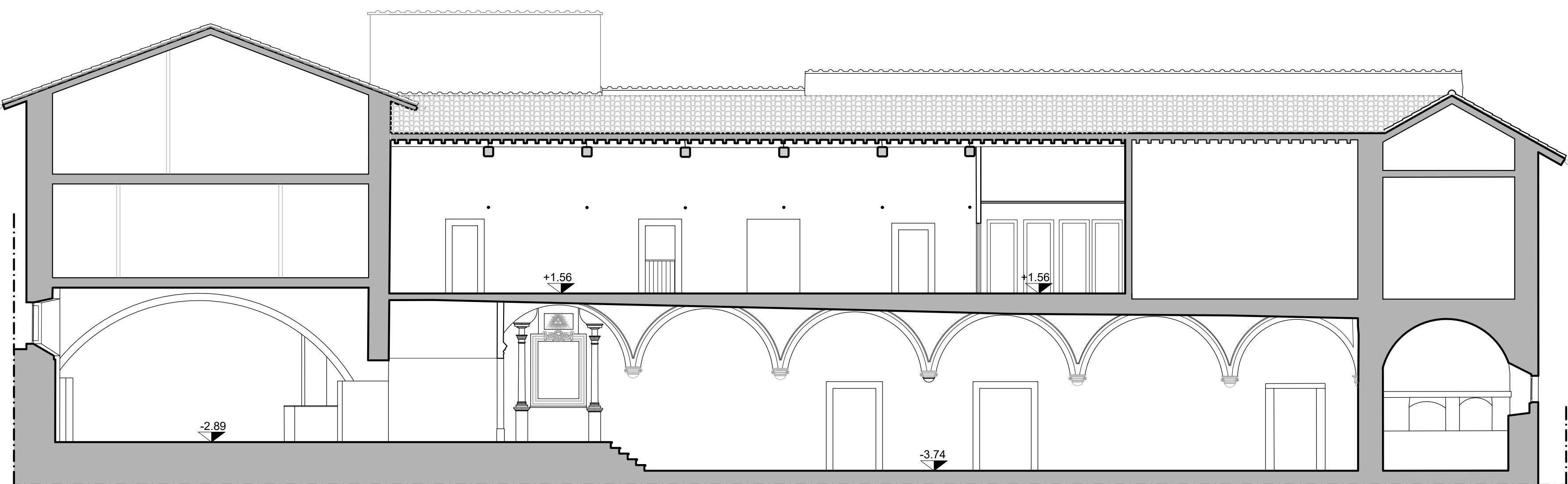
SEZIONE
