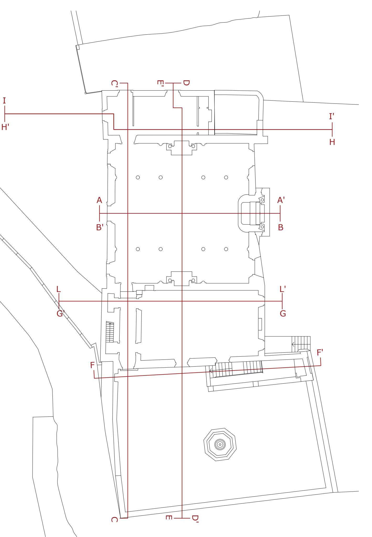
Kplan Planimetria Livello 0 - scala 1:200
