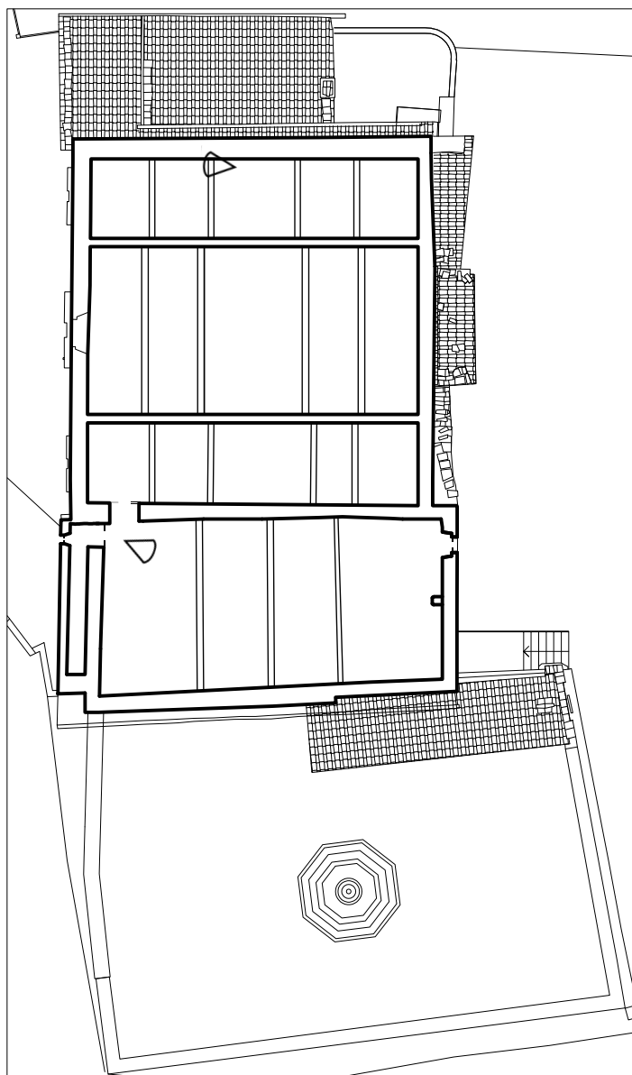
Planimetria Sottotetto
