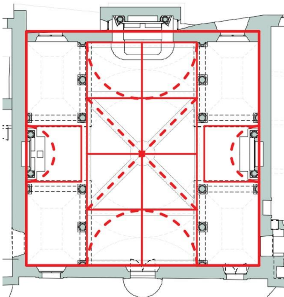
Figura 4 - Schema costruttivo dell'impianto planimetrico
