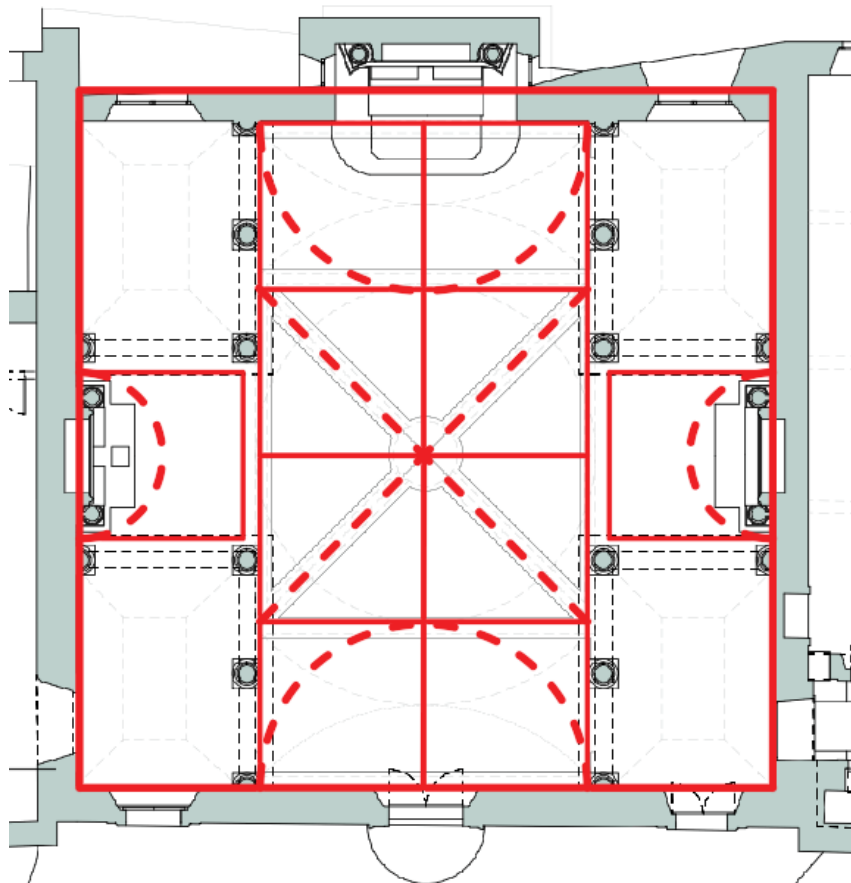
Figura 10 - Schema geometrico della pianta
