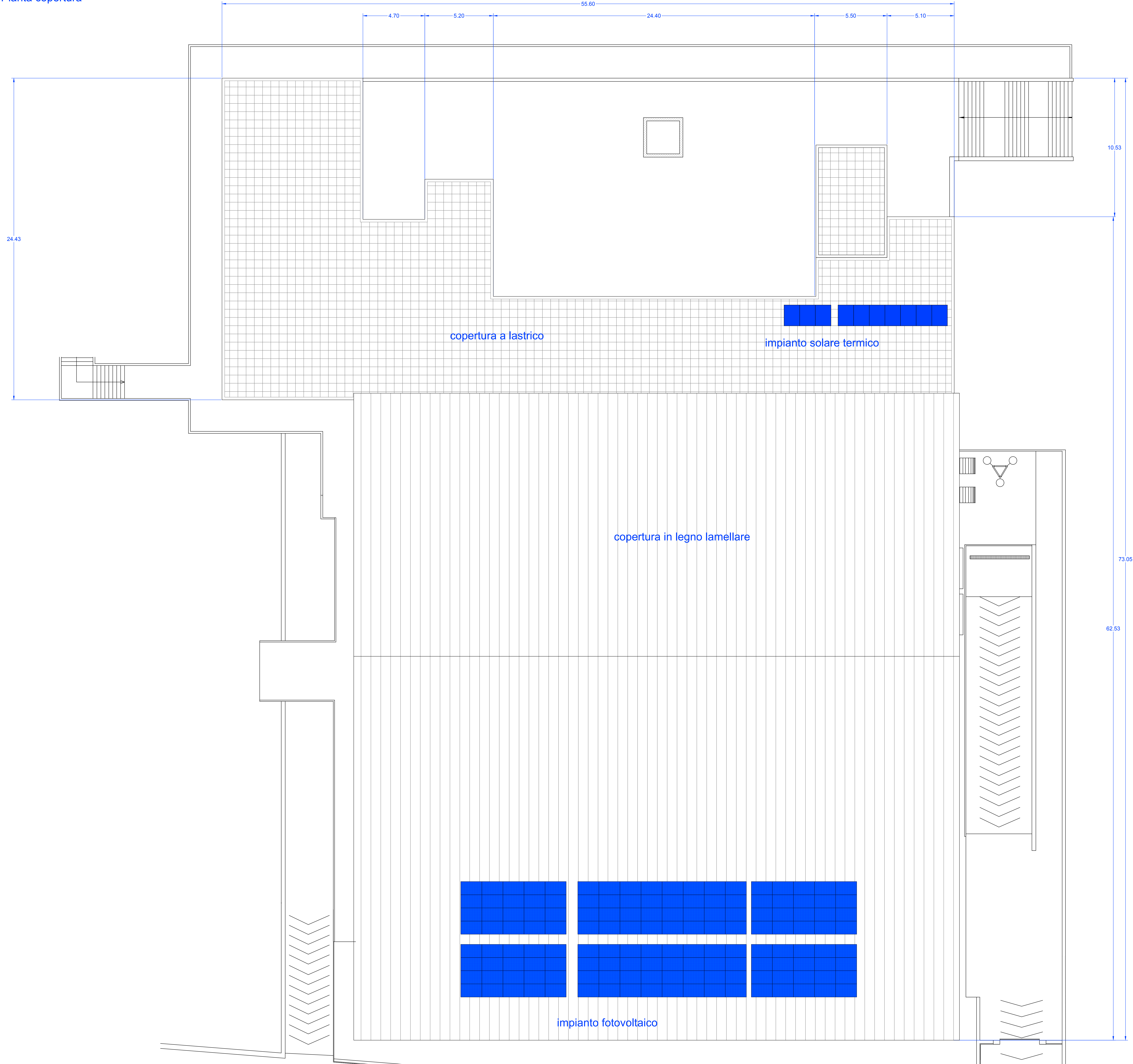
Pianta copertura
